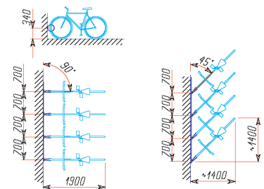
Typ/type KS Serienklammern für Wandmontage Pince en série pour montage mural
